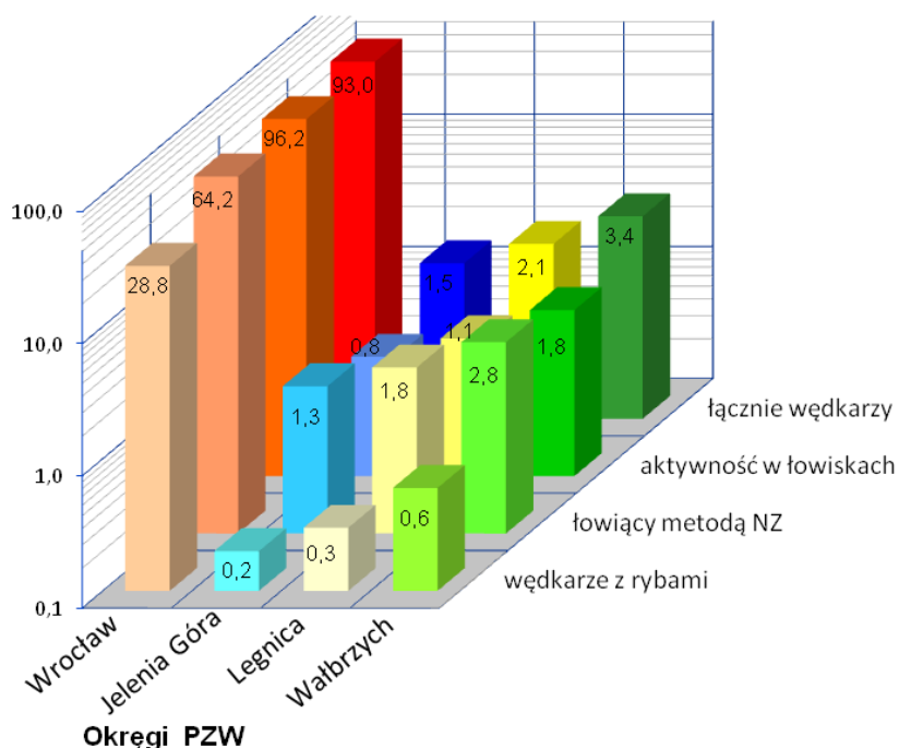
Rys 45 Procentowe oszacowanie ilości i aktywności wrocławskich wędkarzy na dolnośląskich łowiskach odniesione odpowiednio do łącznej liczby wędkarzy (100%) i łącznej aktywności (100%). Wykres wykonano w skali logarytmicznej.
