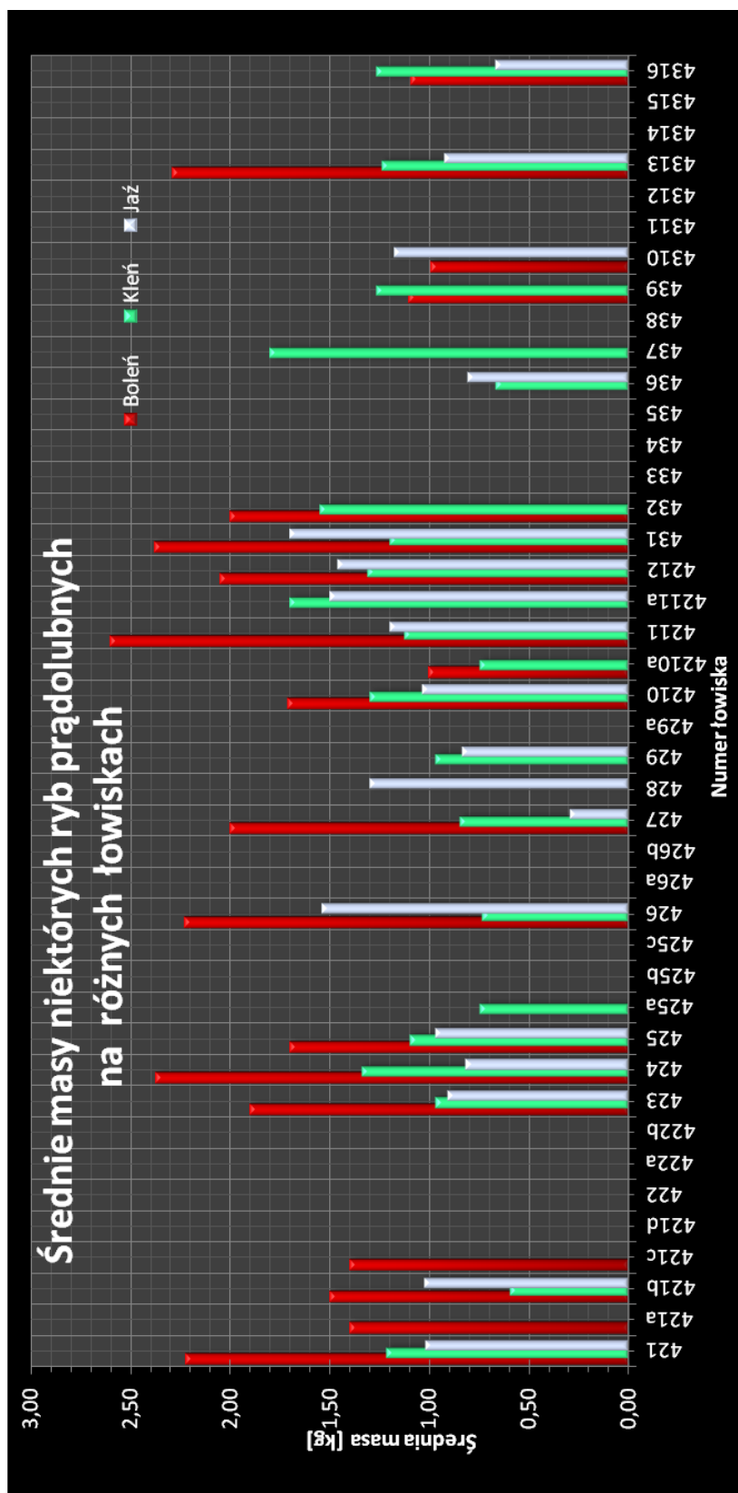
Rys. 48 Średnie masy ryb prądocubnych, które łowiono na różnych łowiskach Okręgu PZW we Wrocławiu
