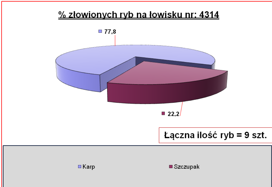
Rys 41 Ilustracja wyników połowów (porządkowanie w kolejności malejącej) opracowana na podstawie: A -masy ryb, B - ilości ryb
